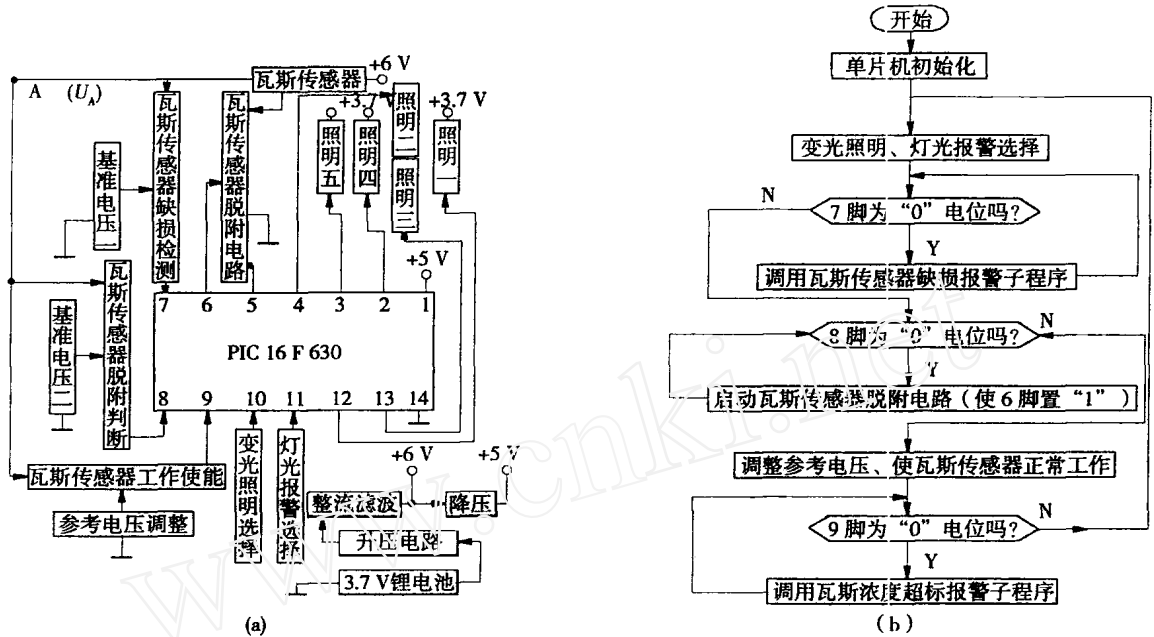
图1 光机电一体化多功能煤矿矿工安全帽控制硬件与主程序框图
